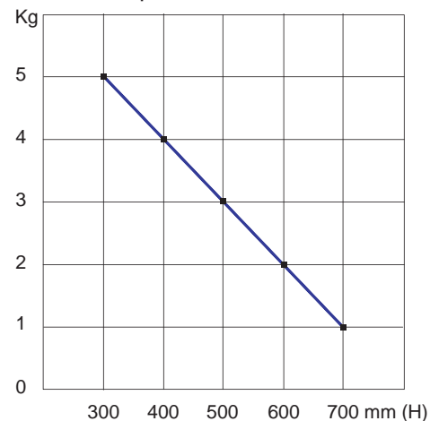
Esempio 1 braccetto 100N*
